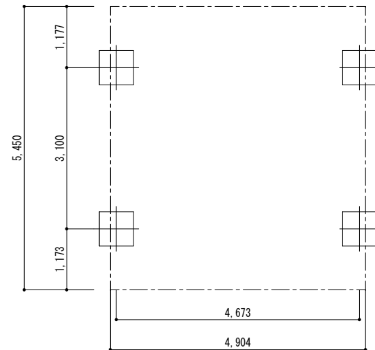
■ 基礎配置図
